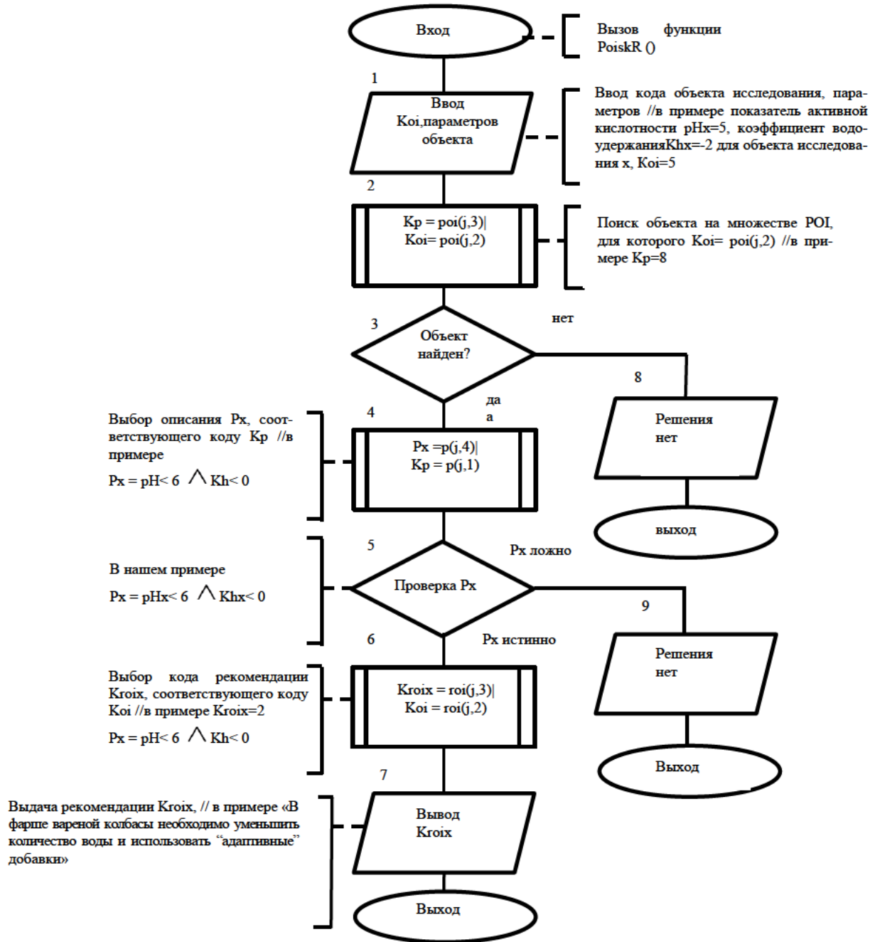
Рисунок 2. Алгоритм работы интеллектуальной (экспертной) системы
