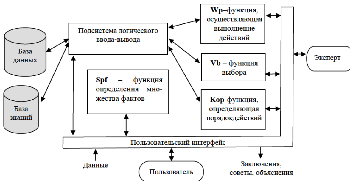
Рисунок1. Типовая структура экспертной системы
